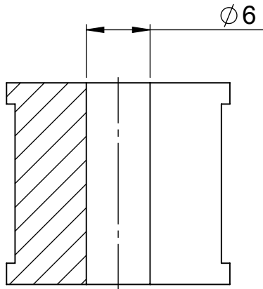
SCHNITT A-A
