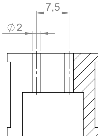
SCHNITT A-A
