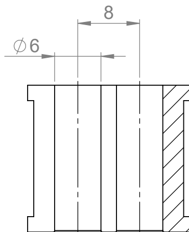
SCHNITT A-A
