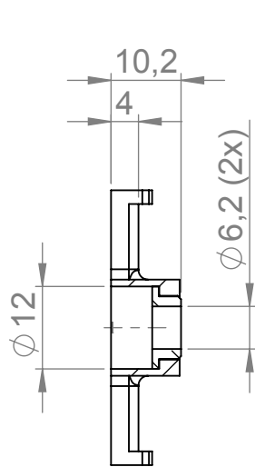
SCHNITT A-A
