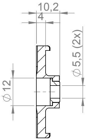
SCHNITT A-A
