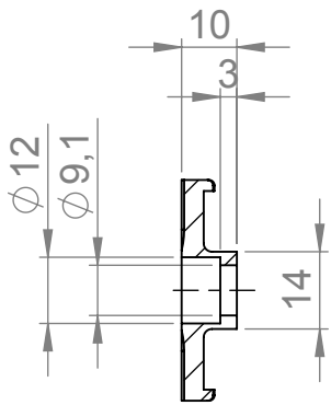
SCHNITT A-A
