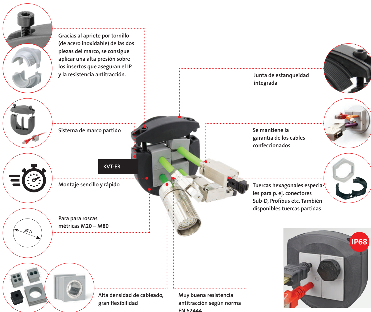
KVT-ER 63/4 con compensador de presión PCE M12x1,5, ver página 100
