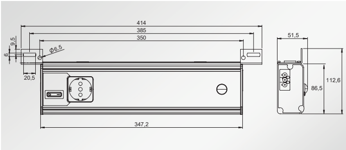
Versión con sensor de movimiento, sin conector para micro de puerta
