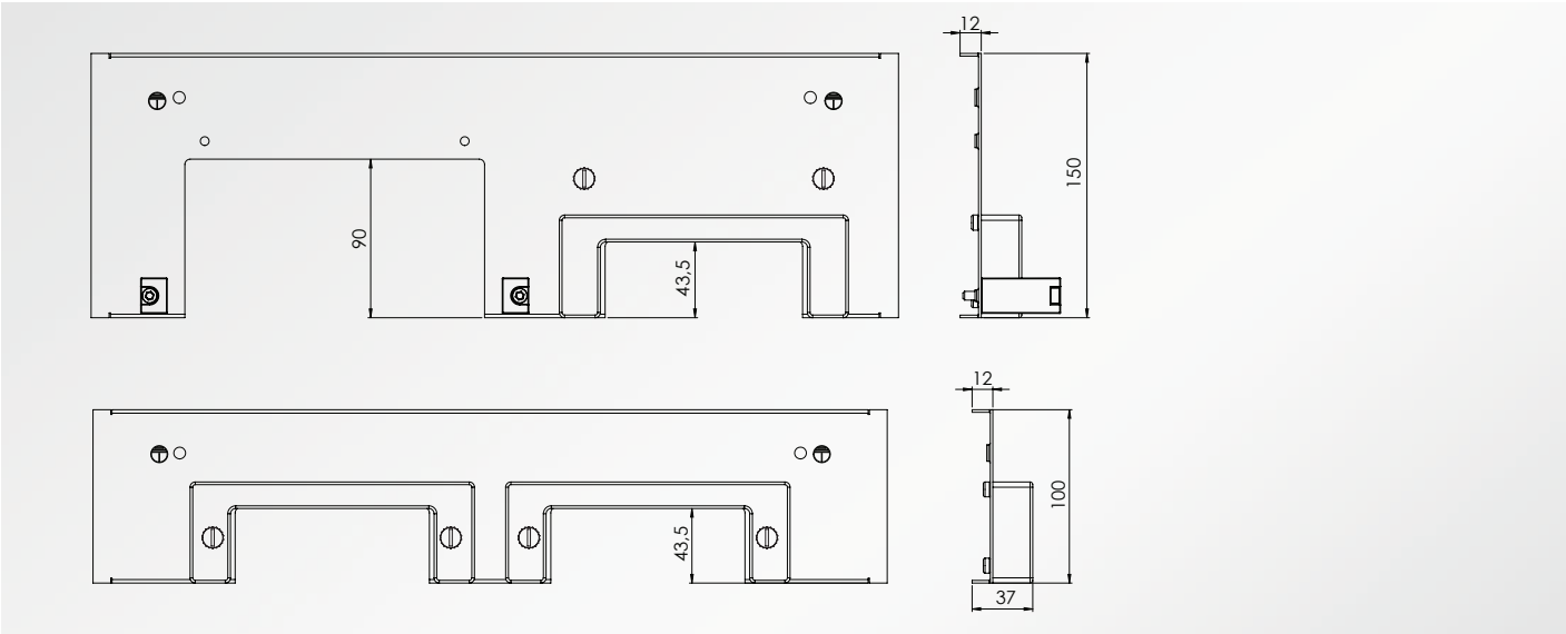
KDR-ESR-TS8 para Rittal TS8
