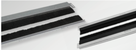
Rittal Placas de suelo con escobillas
