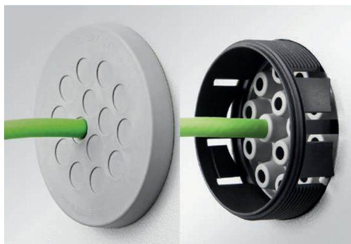
Montaje tipo 1: Encajado en el recorte Para espesores de chapa entre 1 – 2,5 mm
