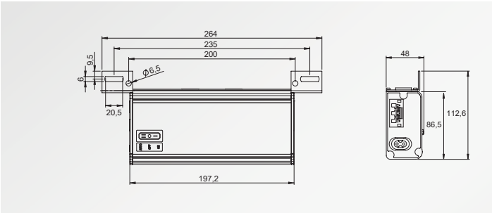
Versión corta sin enchufe US, con conector para interruptor de puerta
