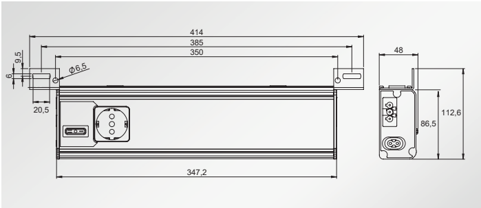
Versión sin sensor de movimiento, con conector para micro de puerta
