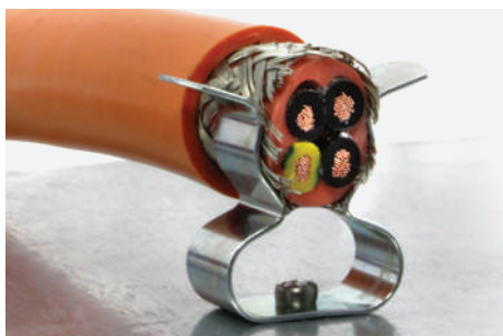
Montaje remachado
