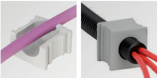
Sección del KTMB
