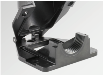
Rosca métrica interna para fijación del tubo
