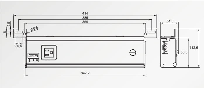
Versión con enchufe US, con sensor de movimiento, sin conector para interruptor de puerta
