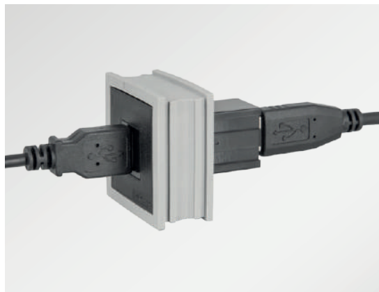
USB (tai RJ45, HDMI) liittimet asennettuna tiivisteosaan. Verkoliittimet painetaan paikalleen sisäpuolelta
