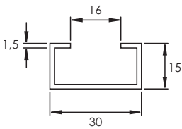
Yhteensopivan C-kiskon mitat (mm)
